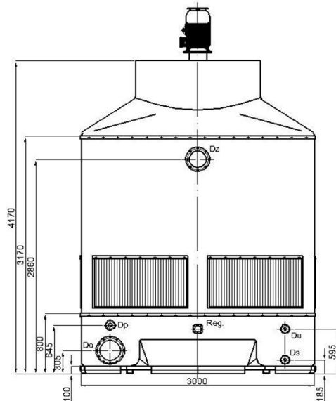
CWT 150/600/SZ
