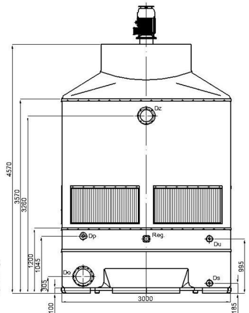
CWT 150/600/PZ
